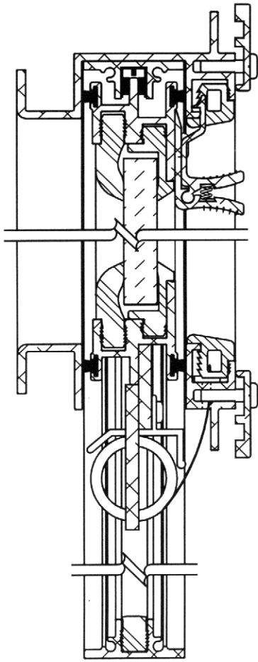
SECTION A-A
